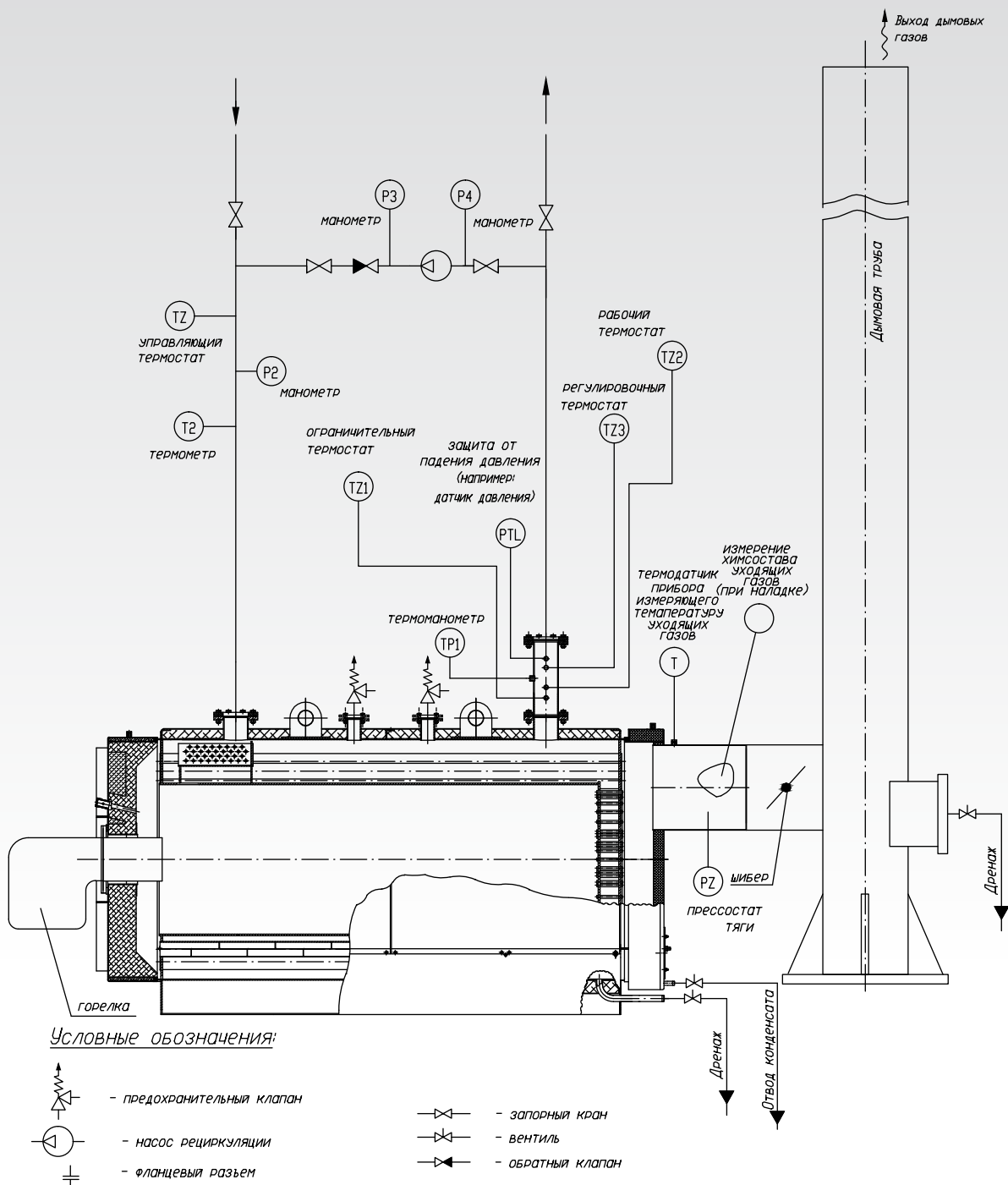
Типовая схема обвязки котла серии ЗИОСАБ
